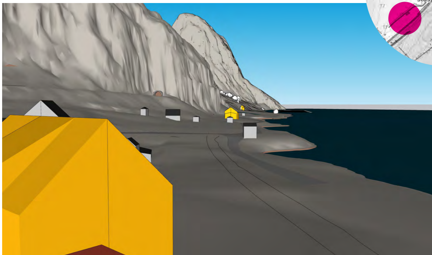
Nullalternativet Ingen endring frå eksisterande situasjon, Bygningar med SEFRAK-verdi er markerte gule og orange, jf. kategori i registeret.
