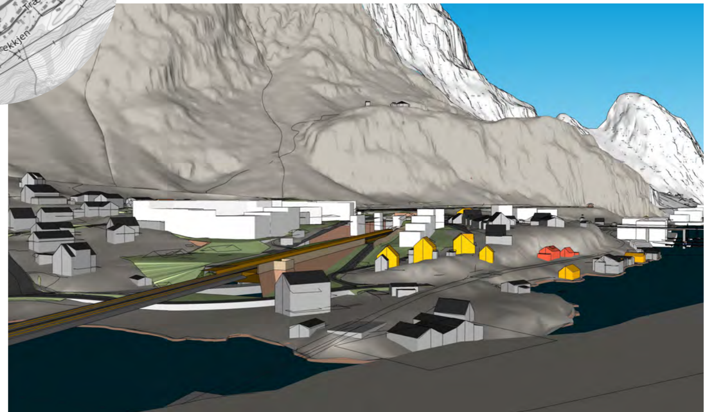
Planforslaget 'litt større' Barnehagebygget er rive og sentrum er omforma heilheitleg
